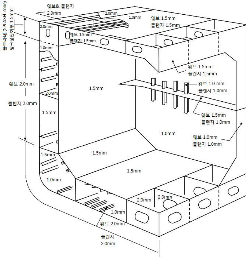
그림 3.1 부식여유
